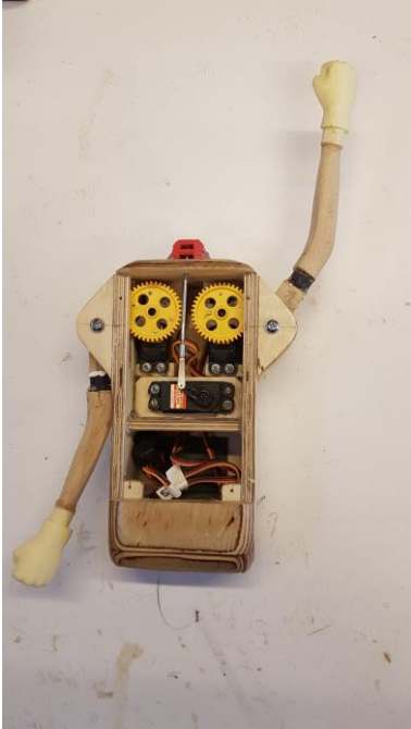
Der fertige Servoeinbau.
